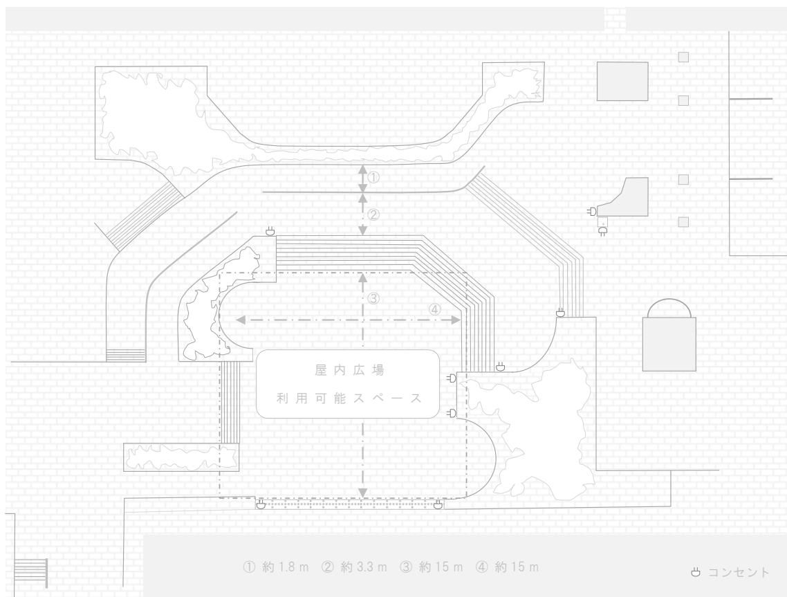
平面図
